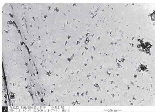
图2 TEM观察AINPs悬浊液经超声处理后的分散情况( \times 120\,000 )
